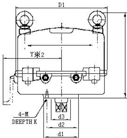
图11 381RSC 型执行器
