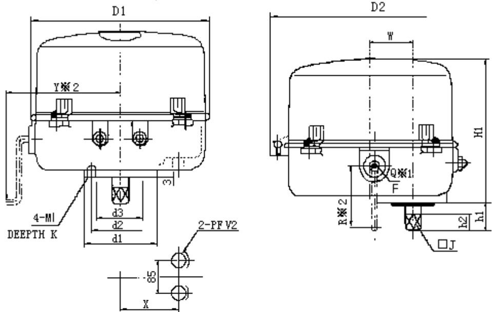
图10 381RSA、381RSB、381RXB 型执行器
