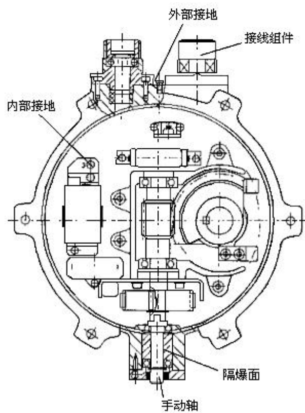
拆卸护罩视图
