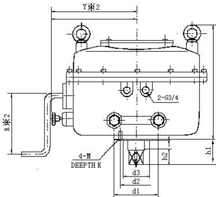
图12 381RSC 型执行器
