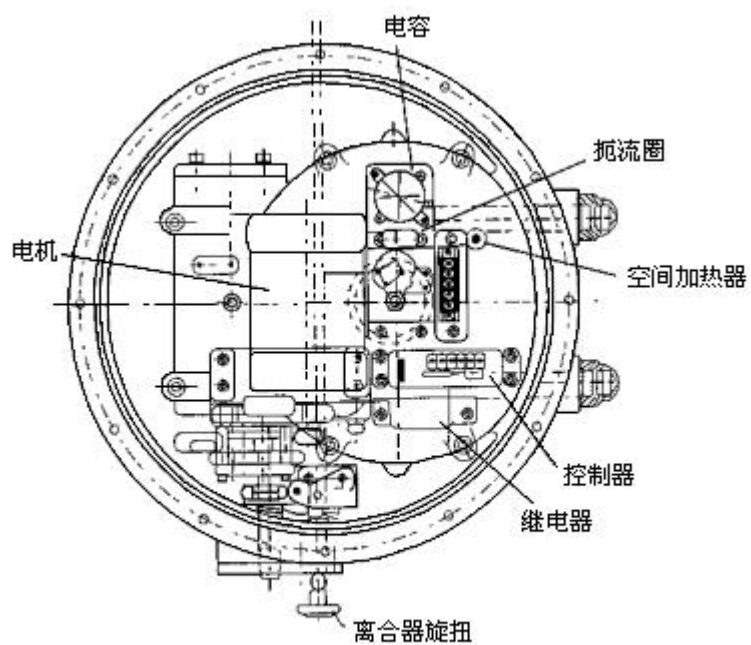
拆卸护罩视图
