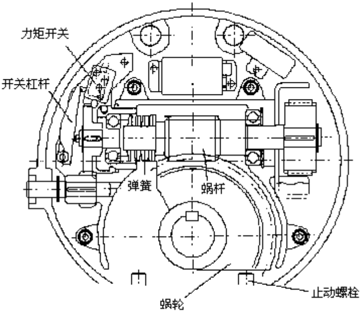
图9 力矩开关动作原理
