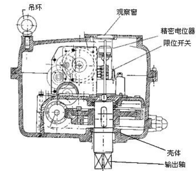
拆卸护罩视图
