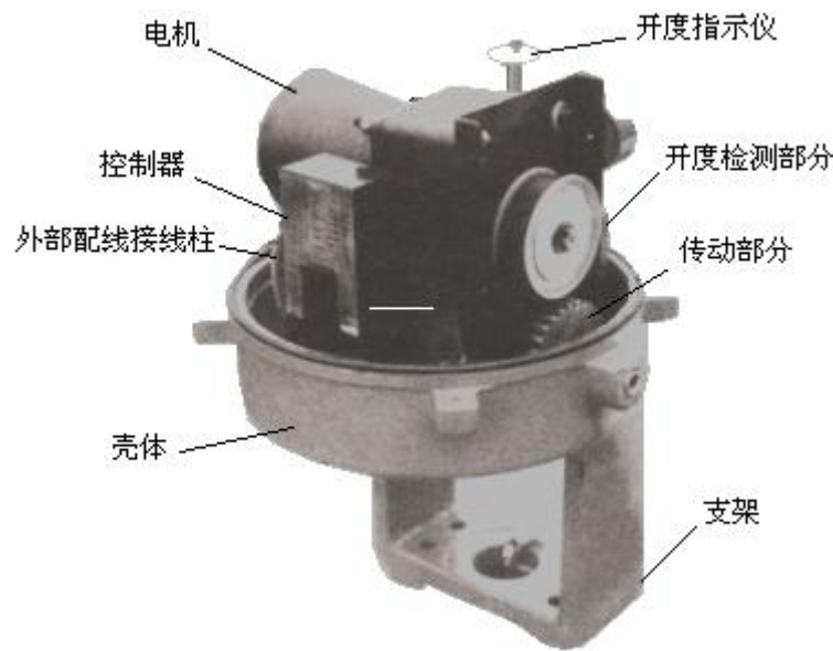
图 1 执行器外观
