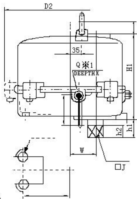
图11 381RSC 型执行器
