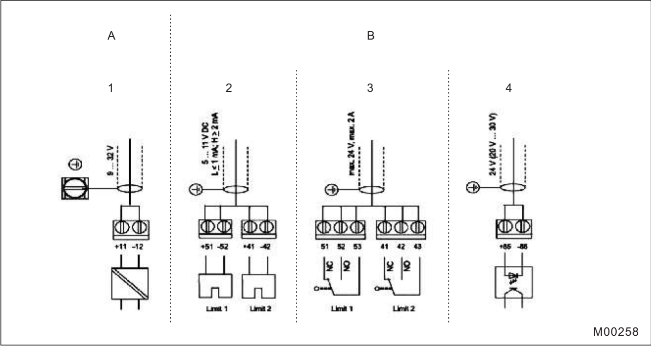
图22 接线配置图
