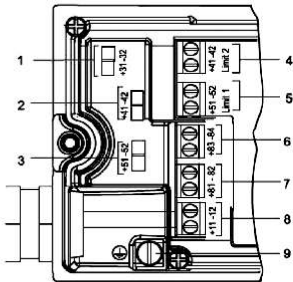
图7 端子分布图
