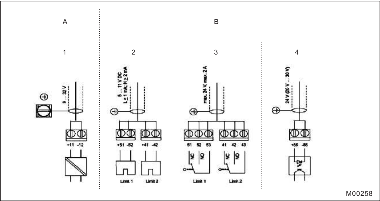
图32 接线配置图
