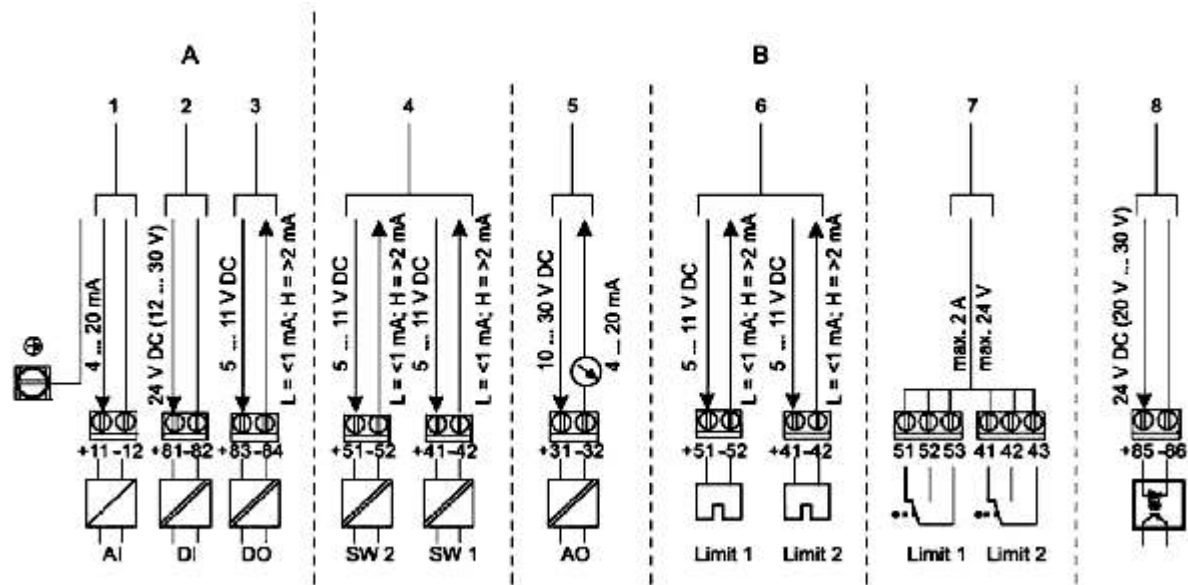
图7 端子分布图
