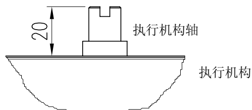
图：执行机构轴的高度(当H=20mm时)
